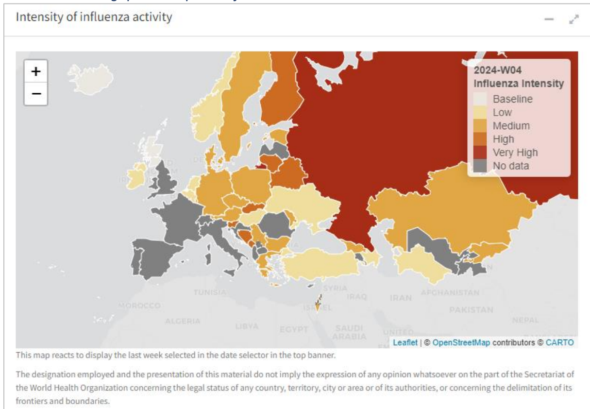
Slika 1. Aktivnost gripe u Europi – 4. Tjedan
