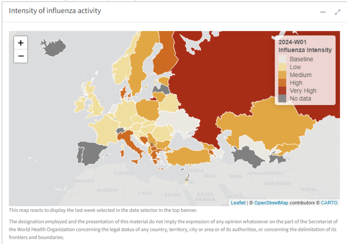
Slika 1. Aktivnost gripe u Europi – 1. Tjedan
